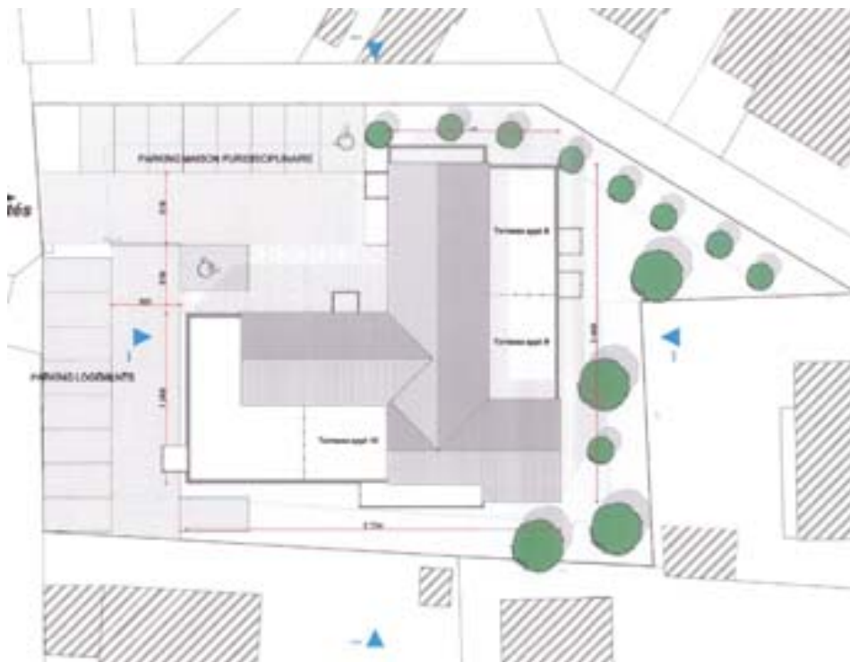
Plan masse du projet
